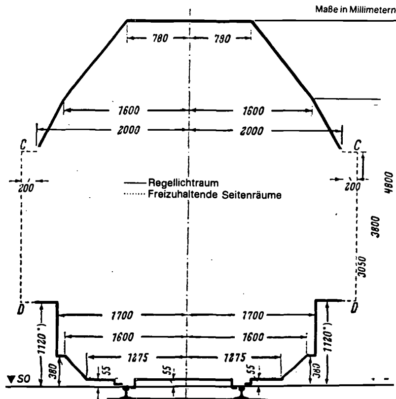
Bild 1 Regellichtraum in der Geraden und in Bögen mit Halbmessern von 250 m und mehr
