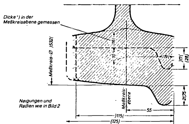
Bild 3 Vollrad
