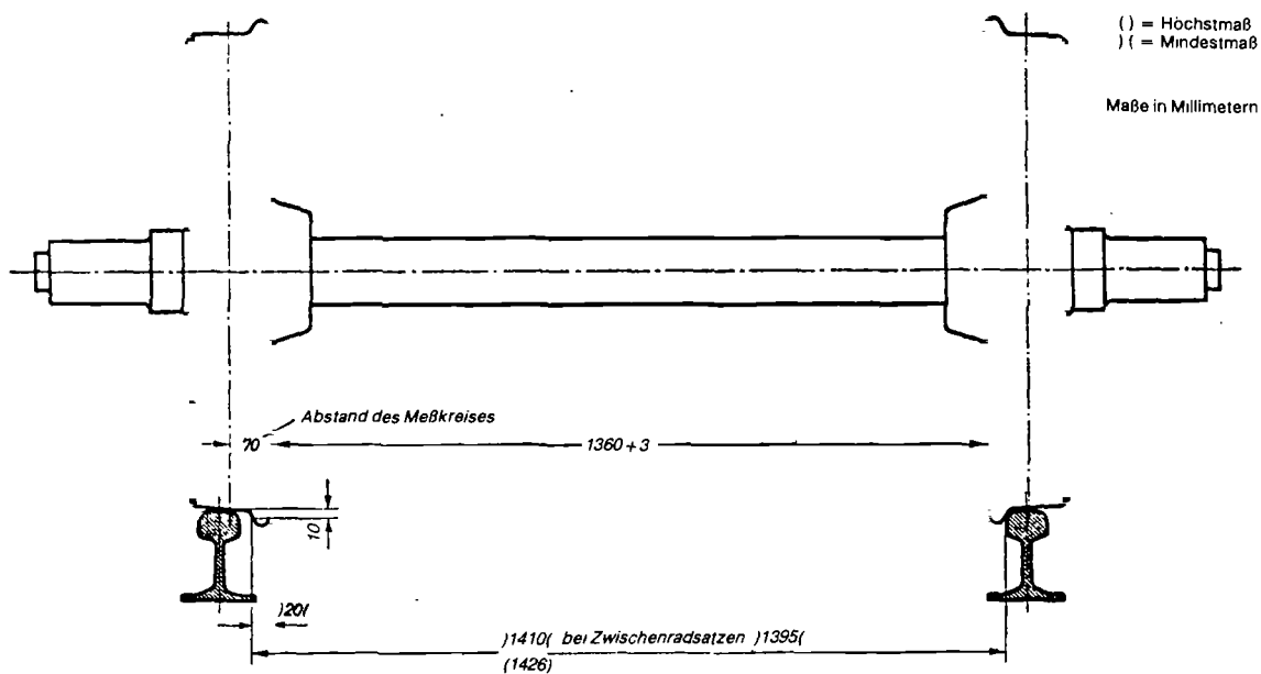
Bild 1 Radsatz
