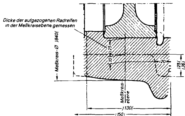
Bild 2 Bereiftes Rad
