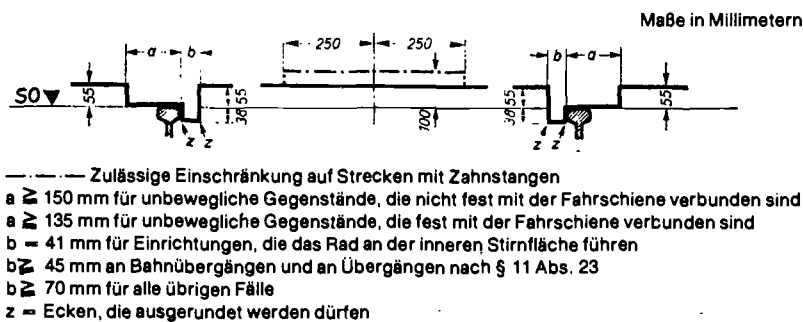
Bild 2 Unterer Teil der Umgrenzung des lichten Raumes
